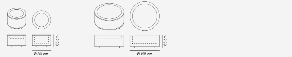
COS 31 A / COS 31 B NET: <17 kg | GROSS: <18 kg
