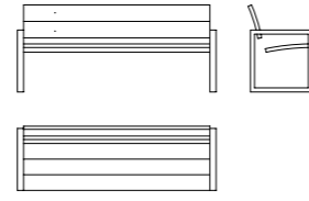
CET 13 192 x 61 x 82 cm NET: <43 | GROSS: <44 kg
